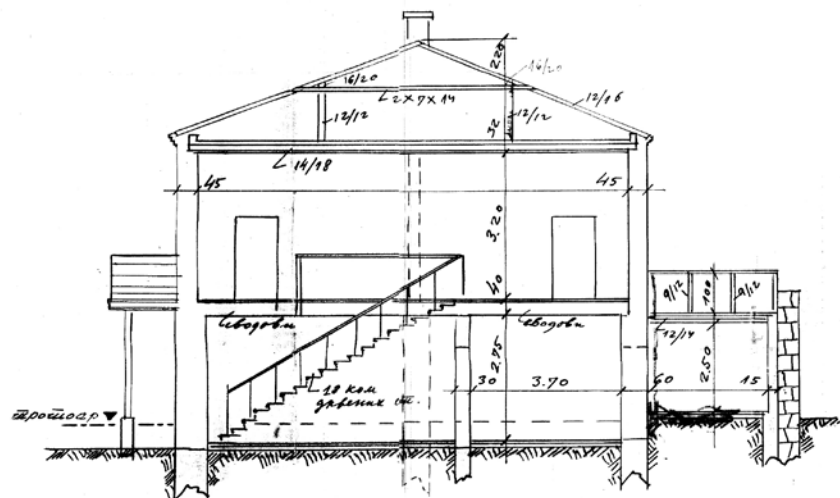
Технички пресек куће урађен 1941. године
